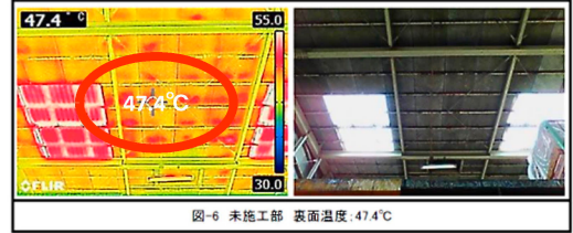
図-6 未施工部 表面温度:47.4°C
