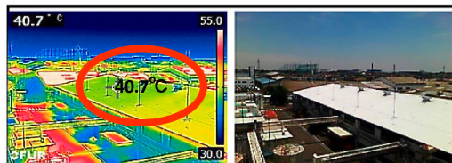
図-2 サーモ遮熱トップ工法(サーモ防水層) 表面温度:40.7°C
